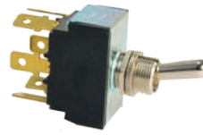
422666 ON/ON DPDT 6 BLADES 25 AMPS 12 VOLT
